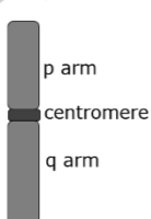
metacentric
